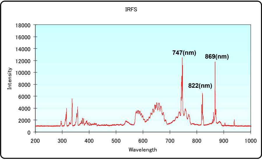
放電スペクトル(窒素) RF電力:300W
